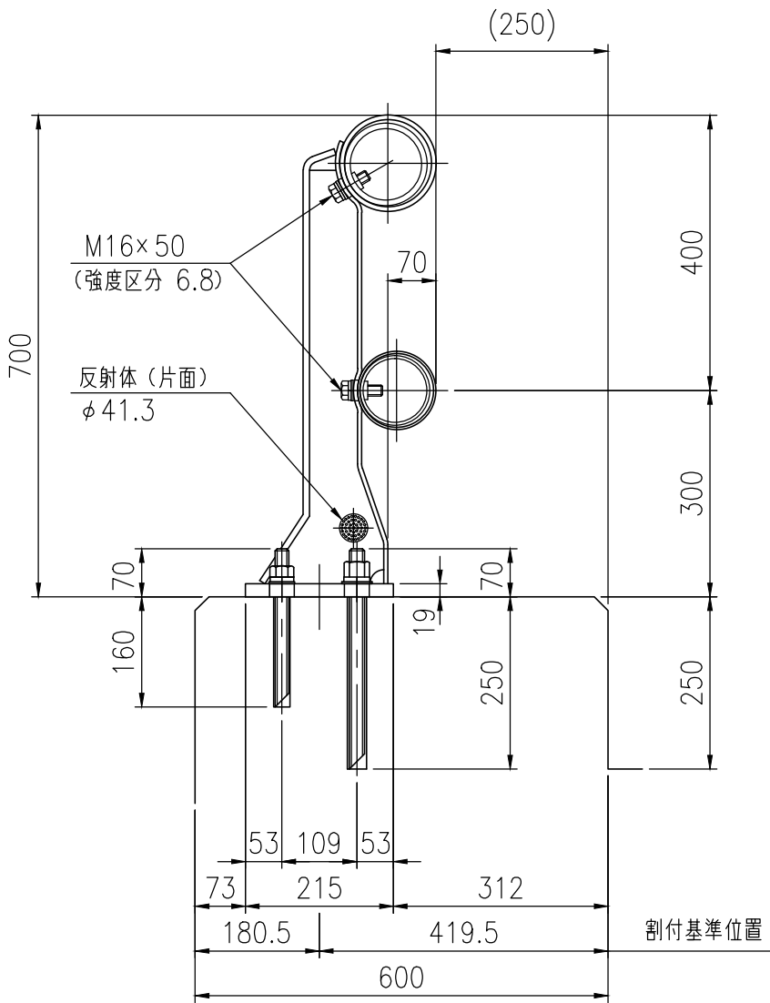
支柱図
