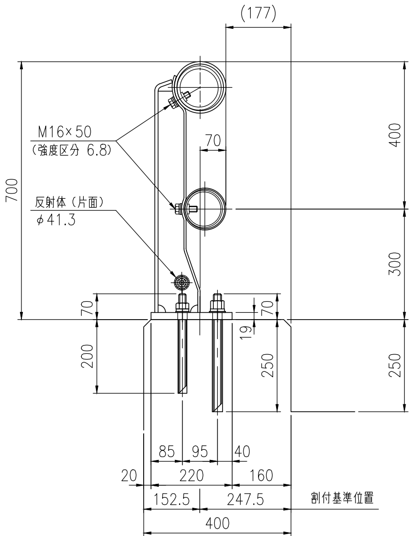
支柱図
