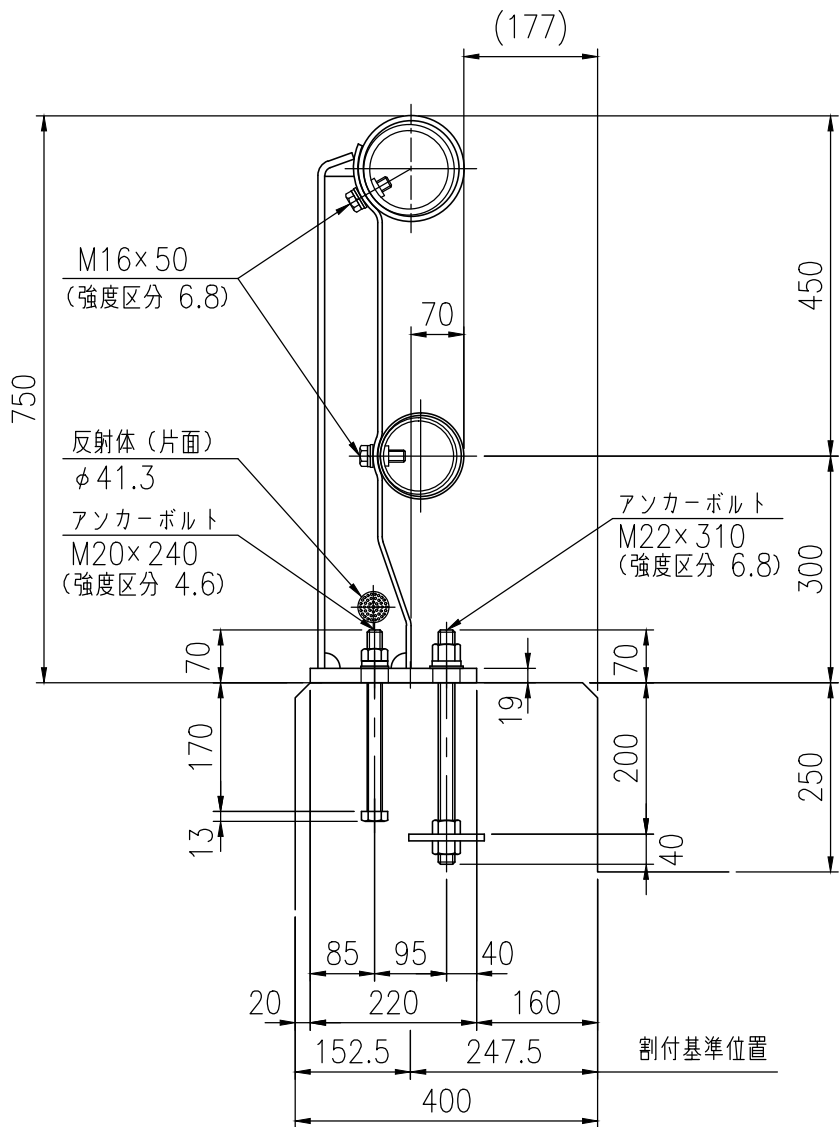
支柱図
