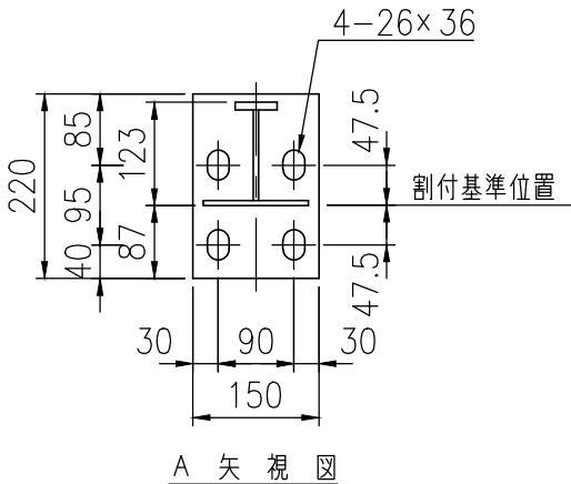
A 矢 視 図
