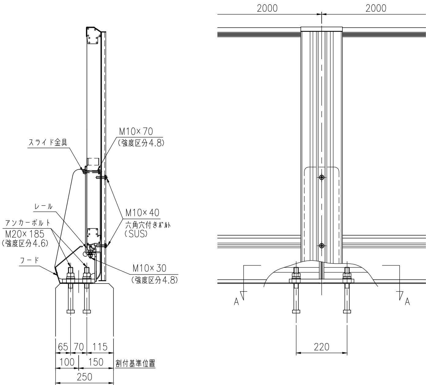
支柱図
