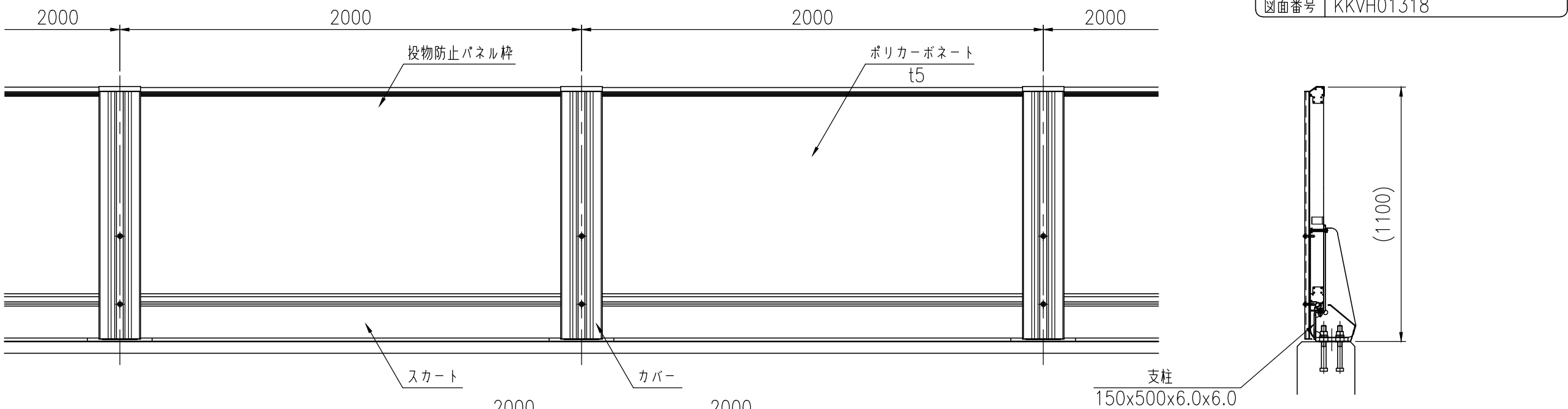
設置図
