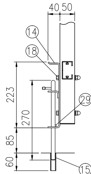
A-A詳細図 (1/8)
