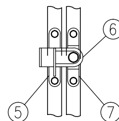
D-D詳細図 (1/8)
