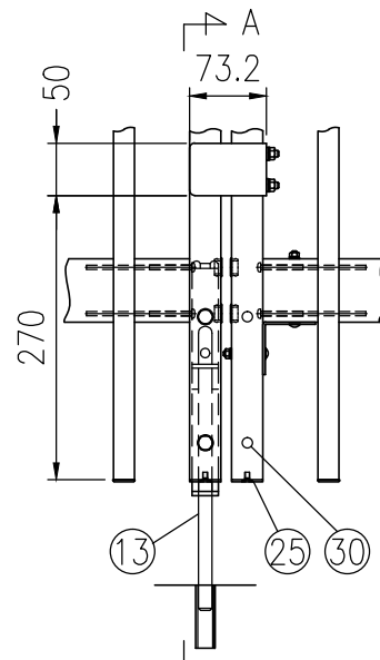
C-C詳細図 (1/8)
