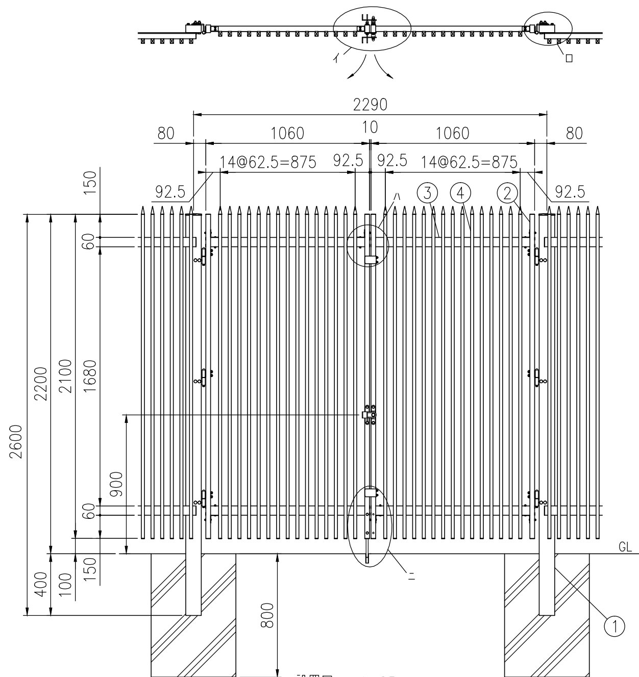
設置図 (1/25) 錠が右、表開きの時 注>基礎の大きさは参考寸法です。
