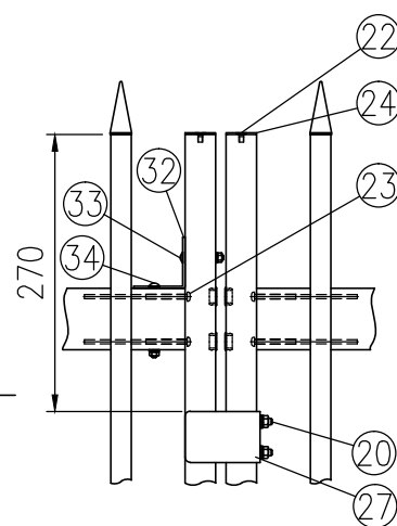
B-B詳細図 (1/8)
