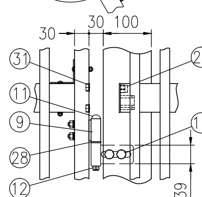
F-F詳細図 (1/8)
