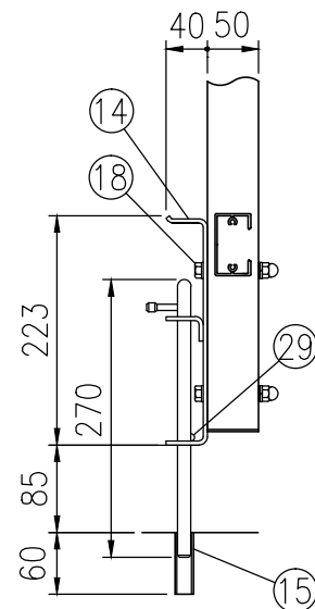
A-A詳細図 (1/8)
