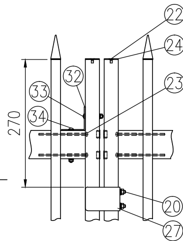
ハ部詳細図 (1/8)
