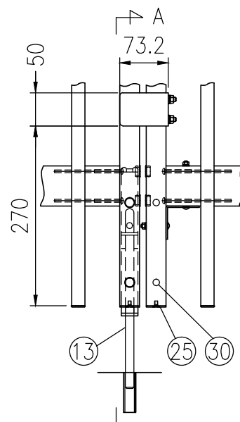
C-C詳細図 (1/8)
