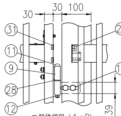
G-G詳細図 (1/8)
