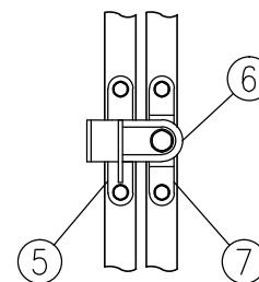
E-E詳細図 (1/8)
