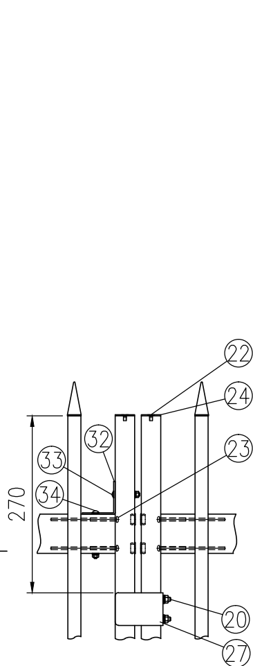
ハ部詳細図 (1/8)
