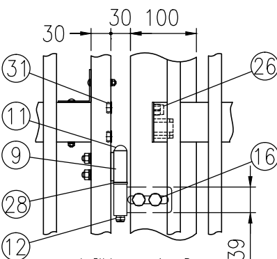
ロ部詳細図 (1/8)
