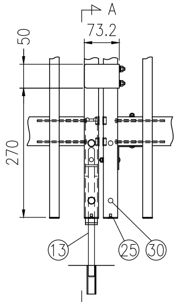
ニ部詳細図 (1/8)
