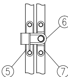
イ部詳細図 (1/8)
