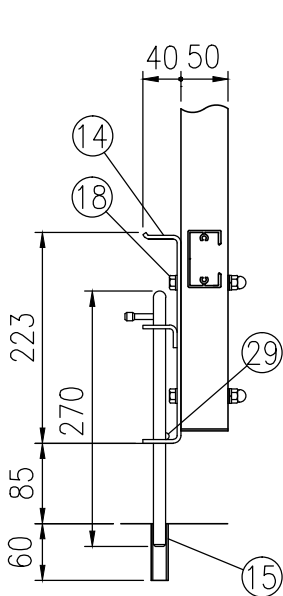
A-A詳細図 (1/8)
