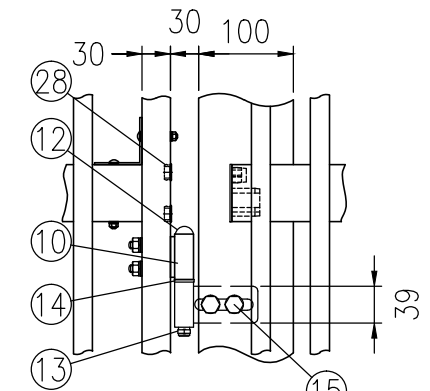
ニ部詳細図 (1/8)
