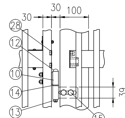
ニ部詳細図 (1/8)
