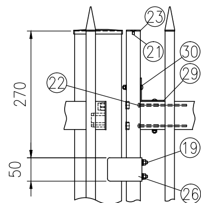
ロ部詳細図 (1/8)
