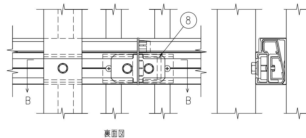
A部 (フェンス接続部) 詳細図 (1/3)
