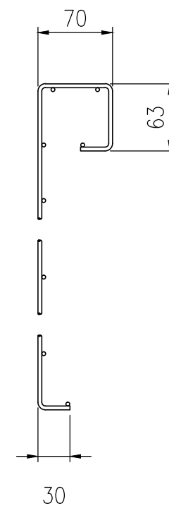
パネル詳細図 (1/5)
