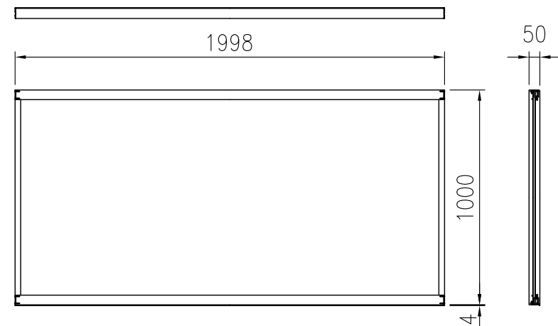
パネル (採光タイプ H1m) 詳細図 (1/25)
