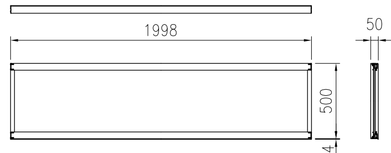
パネル (採光タイプ H0.5m) 詳細図 (1/25)
