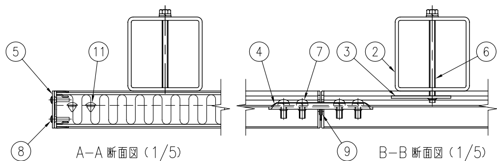
C部 詳細図 (1/5)
