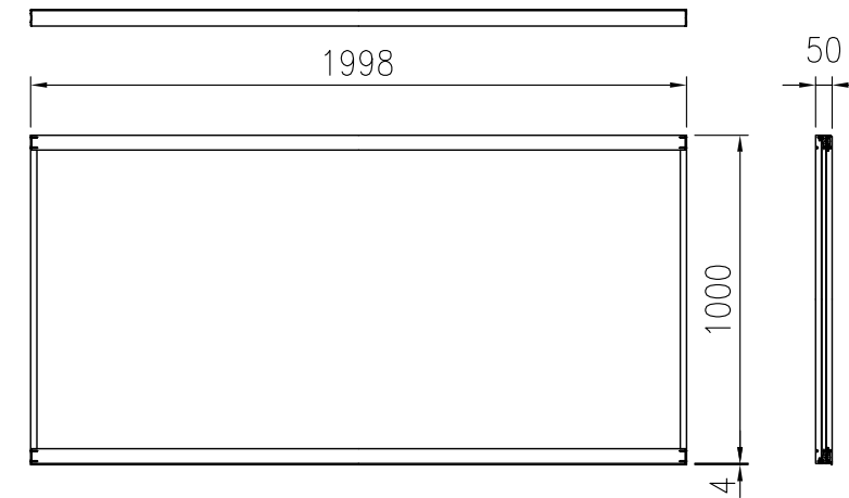
パネル (遮音タイプ H1m) 詳細図 (1/25)
