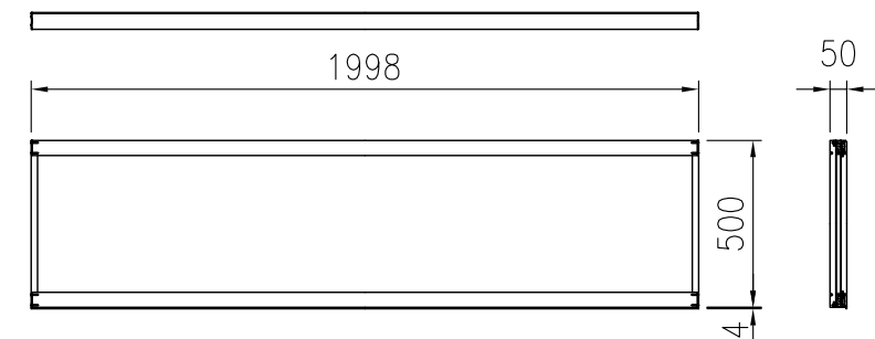
パネル (遮音タイプ H0.5m) 詳細図 (1/25)
