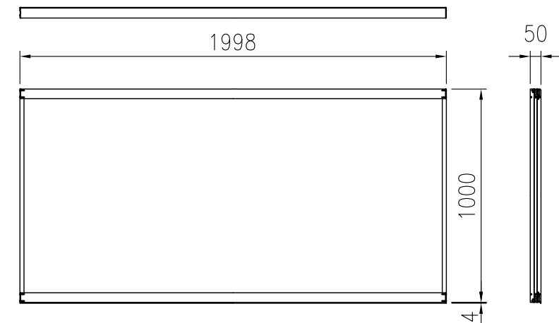
パネル (遮音タイプ H1m) 詳細図 (1/25)
