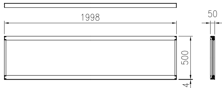
パネル (遮音タイプ H0.5m) 詳細図 (1/25)
