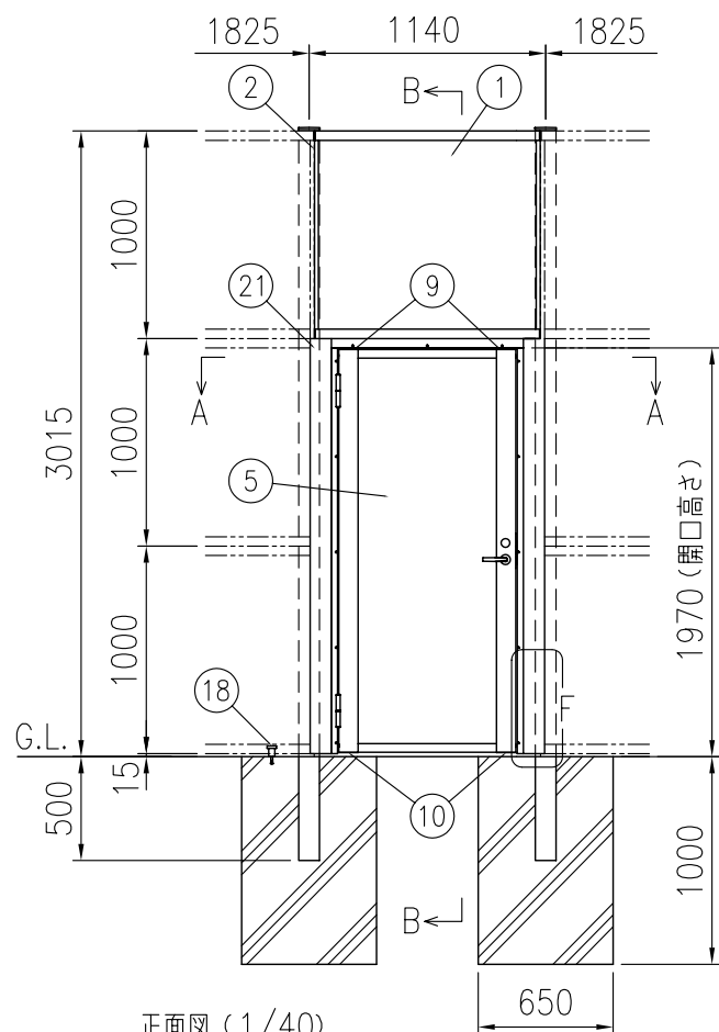
正面図 (1/40)
