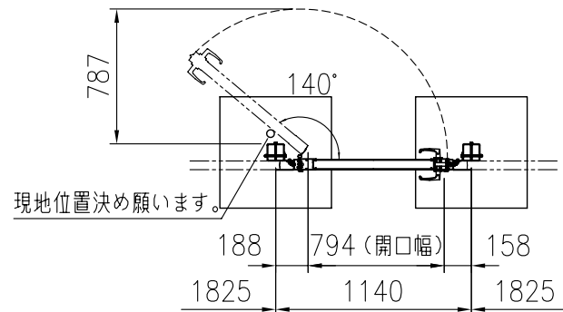
A-A 断面図 (1/40) 逆開きの場合
