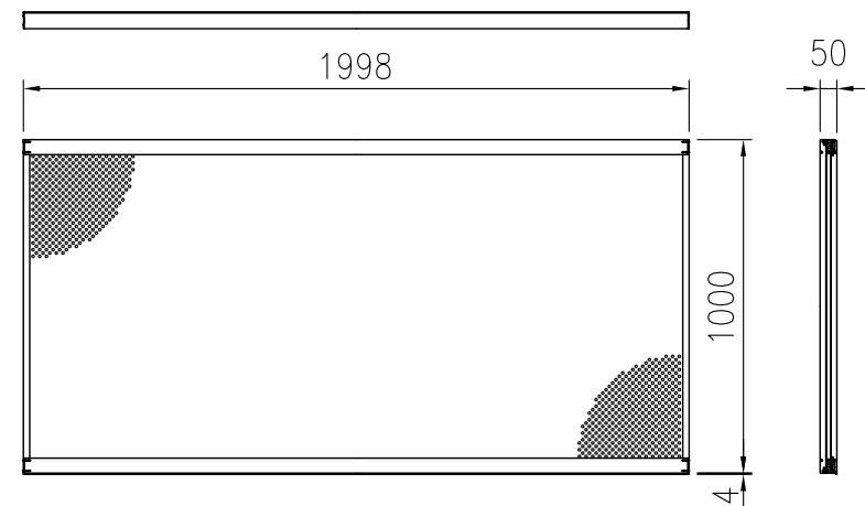
パネル (吸音タイプ H1m) 詳細図 (1/25)
