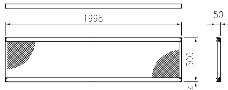
パネル (吸音タイプ H0.5m) 詳細図 (1/25)
