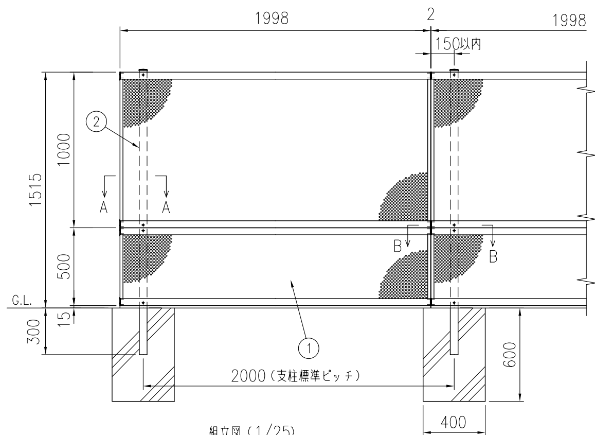
組立図 (1/25)
