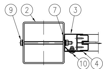
C-C 断面図 (1/8)
