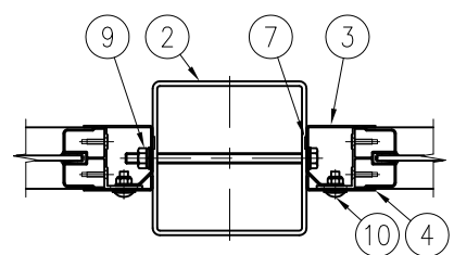
D-D 断面図 (1/8)
