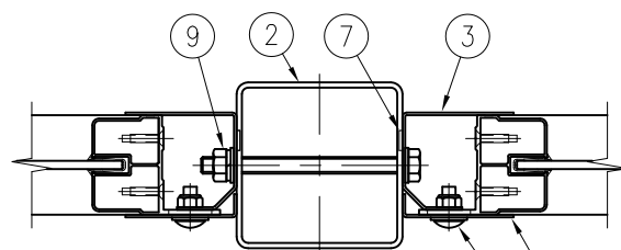
D-D 断面図 (1/5)
