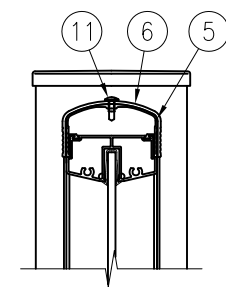
E部 詳細図 (1/5)
