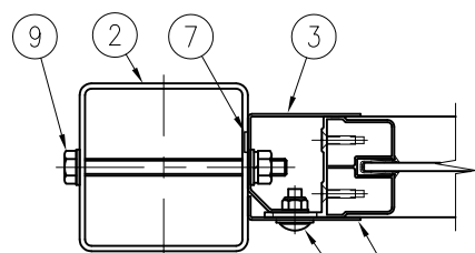
C-C 断面図 (1/5)
