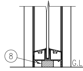
F部 詳細図 (1/5)
