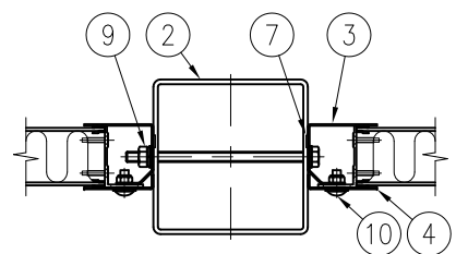
D-D 断面図 (1/8)
