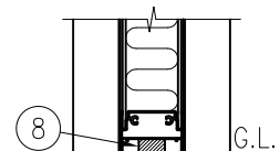
F部 詳細図 (1/8)
