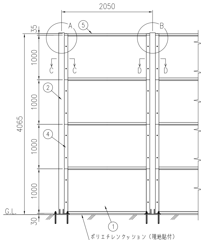
組立図 (1/40)
