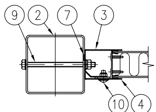
C-C 断面図 (1/8)
