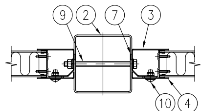
D-D 断面図 (1/8)
