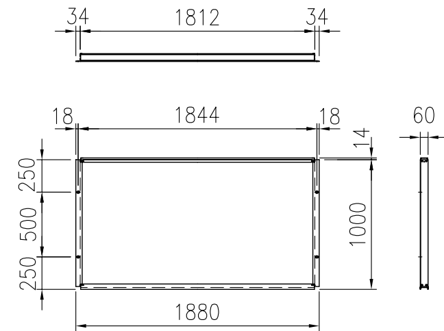
パネル (遮音タイプ H1m) 詳細図 (1/40)
