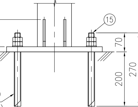
ベースプレート詳細図 (1/8)
