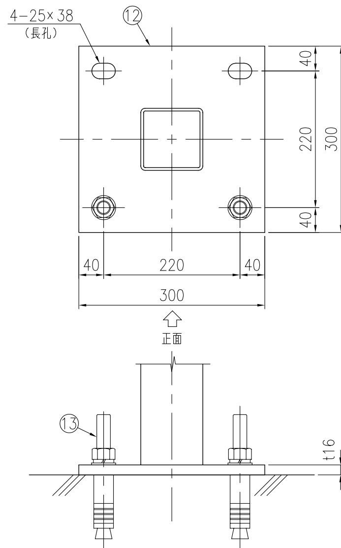
ベースプレート詳細図 (1/6)
