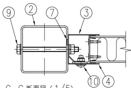
C-C 断面図 (1/5)
