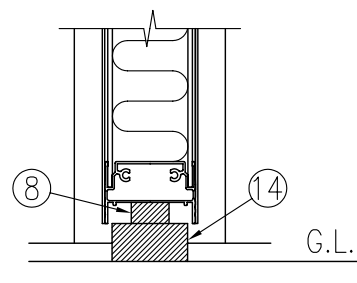
F部 詳細図 (1/5)
