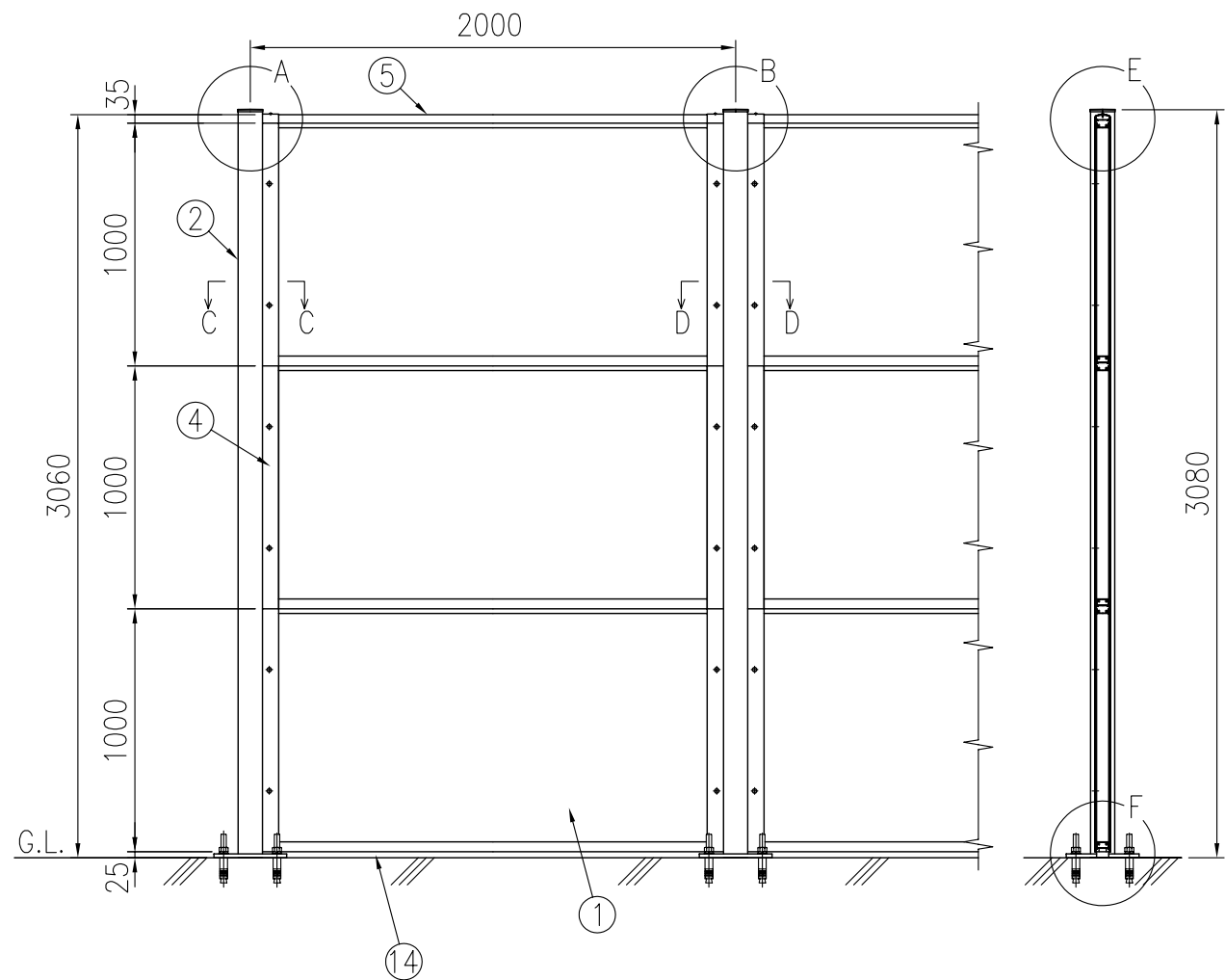
組立図 (1/30)
