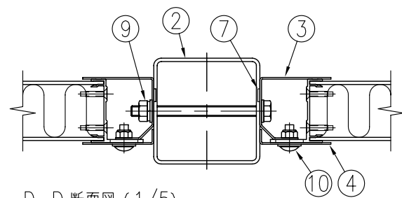
D-D 断面図 (1/5)
