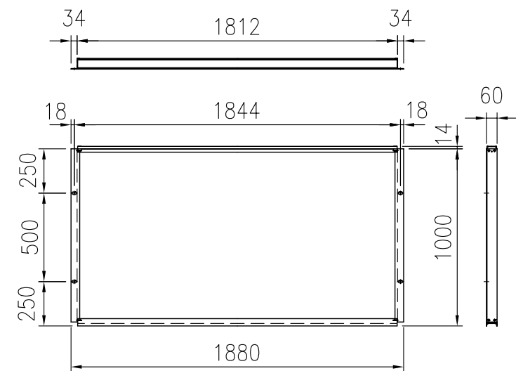
パネル (遮音タイプ H1m) 詳細図 (1/30)
