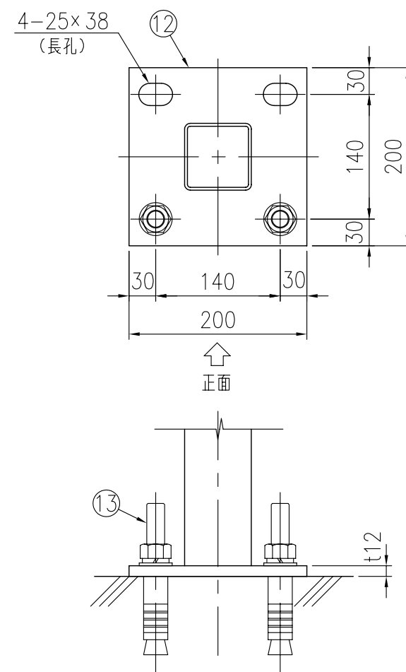
ベースプレート詳細図 (1/6)
