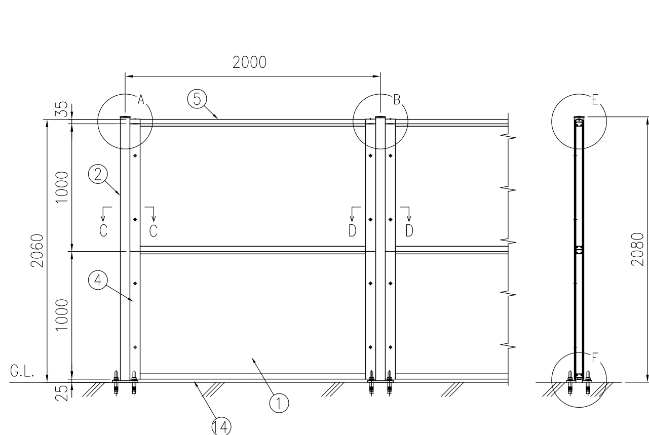
組立図 (1/30)
