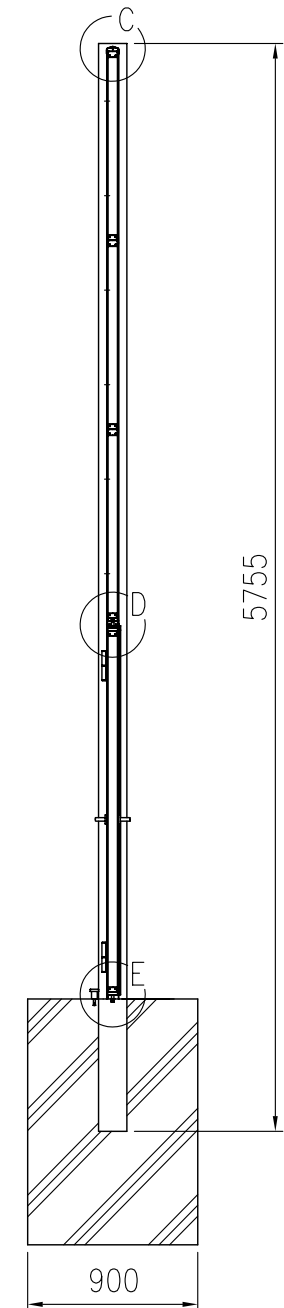
B-B 断面図 (1/40)
