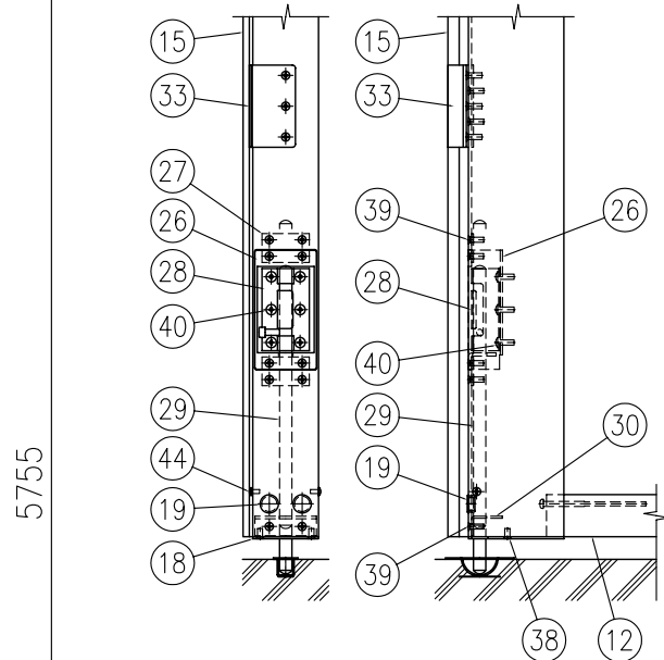
F部側面詳細図 (1/8) F部詳細図 (1/8) ※門扉パネル(受側)のF部とC部は上下対称
