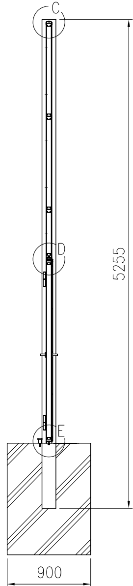
B-B 断面図 (1/40)
