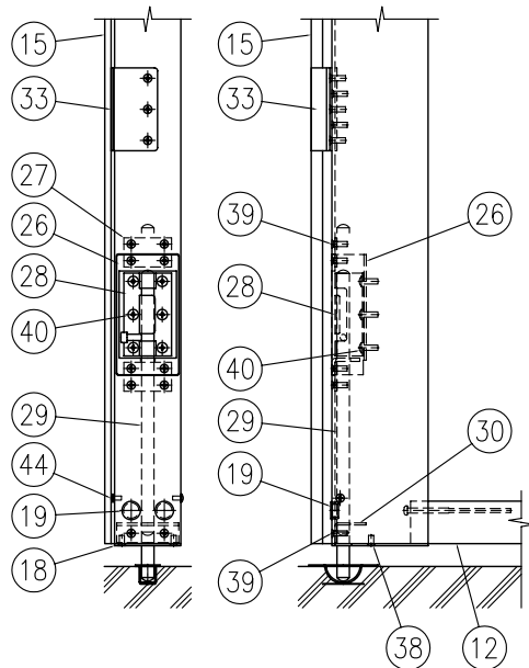
F部側面詳細図 (1/8) F部詳細図 (1/8) ※門扉パネル(受側)のF部とC部は上下対称
