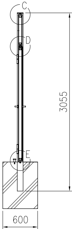
B-B 断面図 (1/40)
