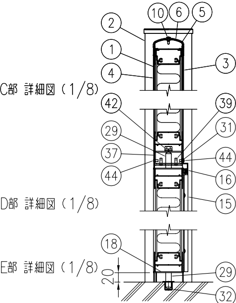
※(32)は門扉パネル取付後、下空寸法 (20)を守って高さ調整して下さい。
