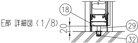
※(32)は門扉パネル取付後、下空寸法 (20)を守って高さ調整して下さい。
