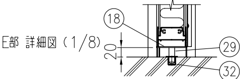
※(32)は門扉パネル取付後、下空寸法 (20)を守って高さ調整して下さい。
