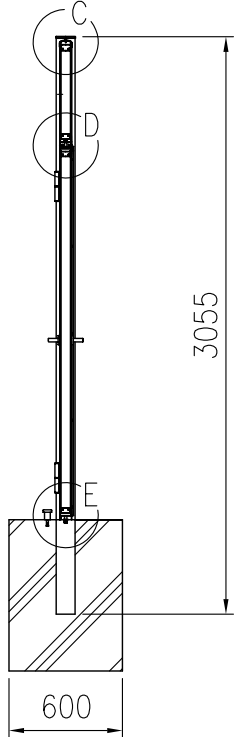
B-B 断面図 (1/40)
