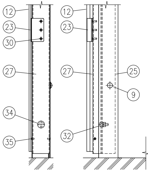
F部側面詳細図 (1/8)
