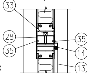
D部 詳細図 (1/8)
