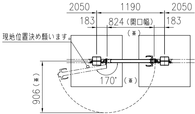
A-A 断面図 (1/40)
