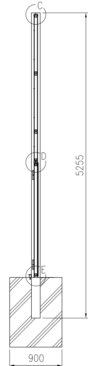
B-B 断面図 (1/40)
