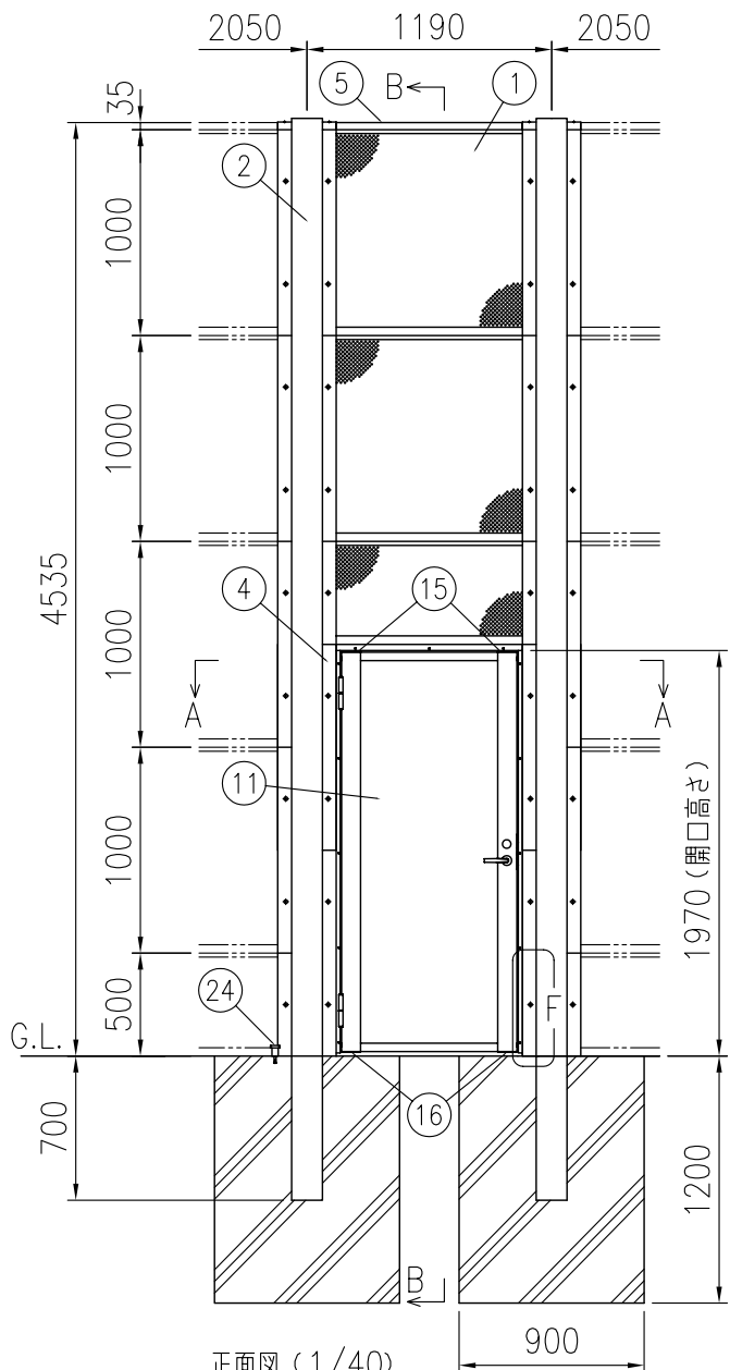
正面図 (1/40)
