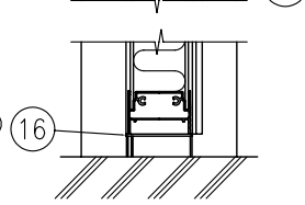
E部 詳細図 (1/8)
