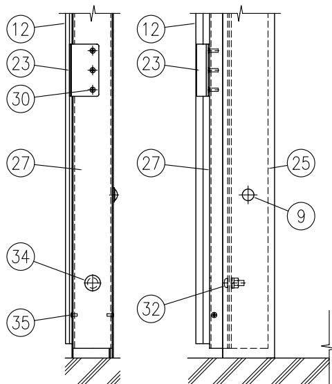
F部側面詳細図 (1/8)
