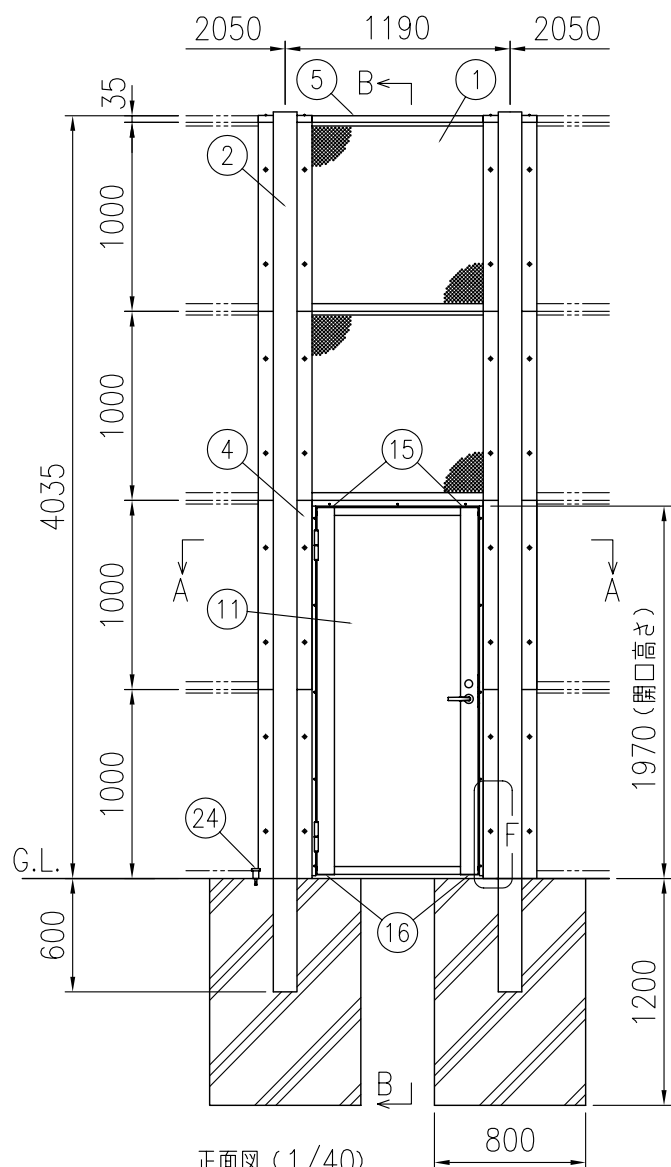
正面図 (1/40)
