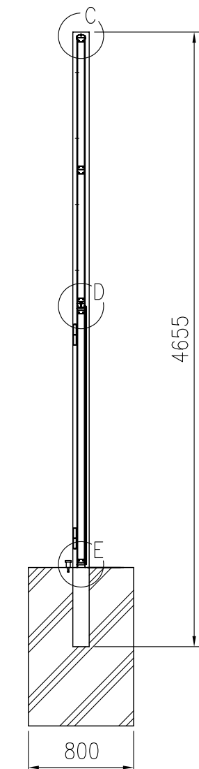
B-B 断面図 (1/40)
