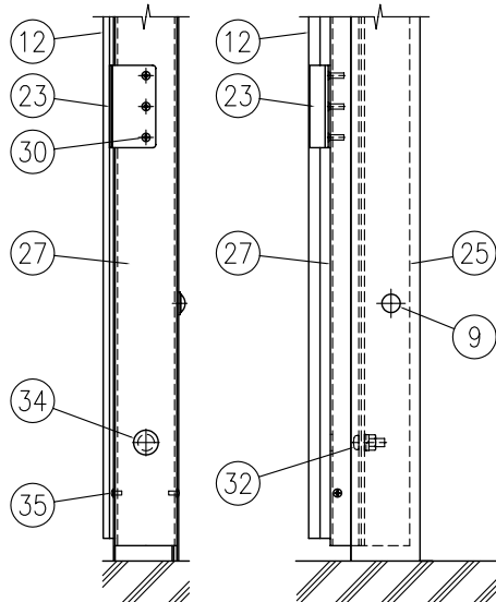
F部側面詳細図 (1/8)
