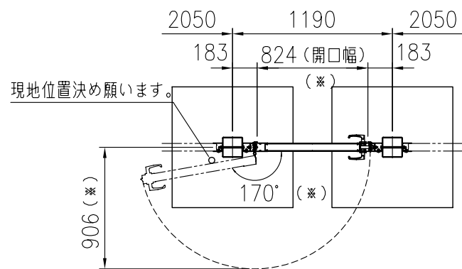
A-A 断面図 (1/40)
