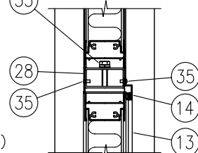
D部 詳細図 (1/8)
