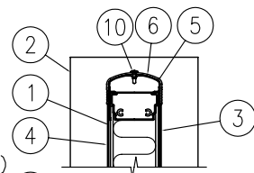
C部 詳細図 (1/8)
