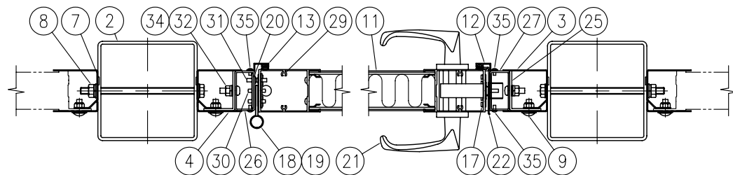
A-A 断面詳細図 (1/8)
