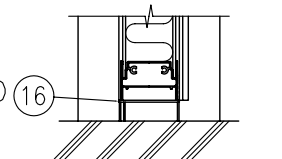
E部 詳細図 (1/8)
