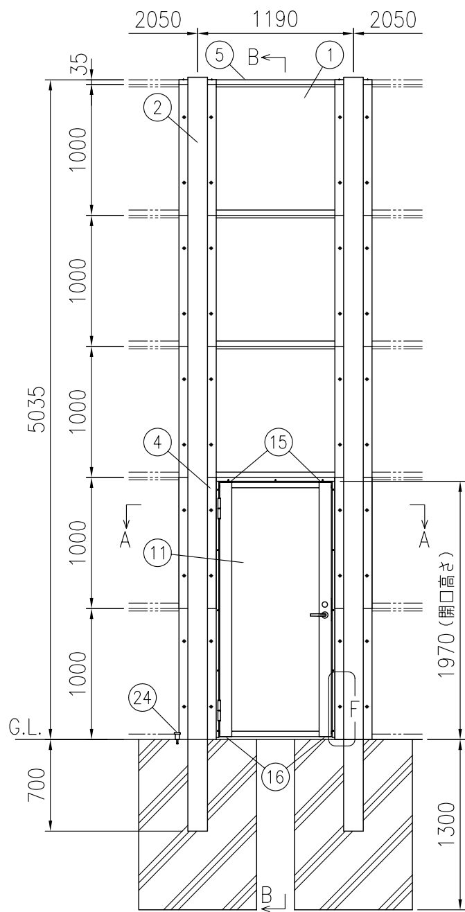
正面図 (1/40)
