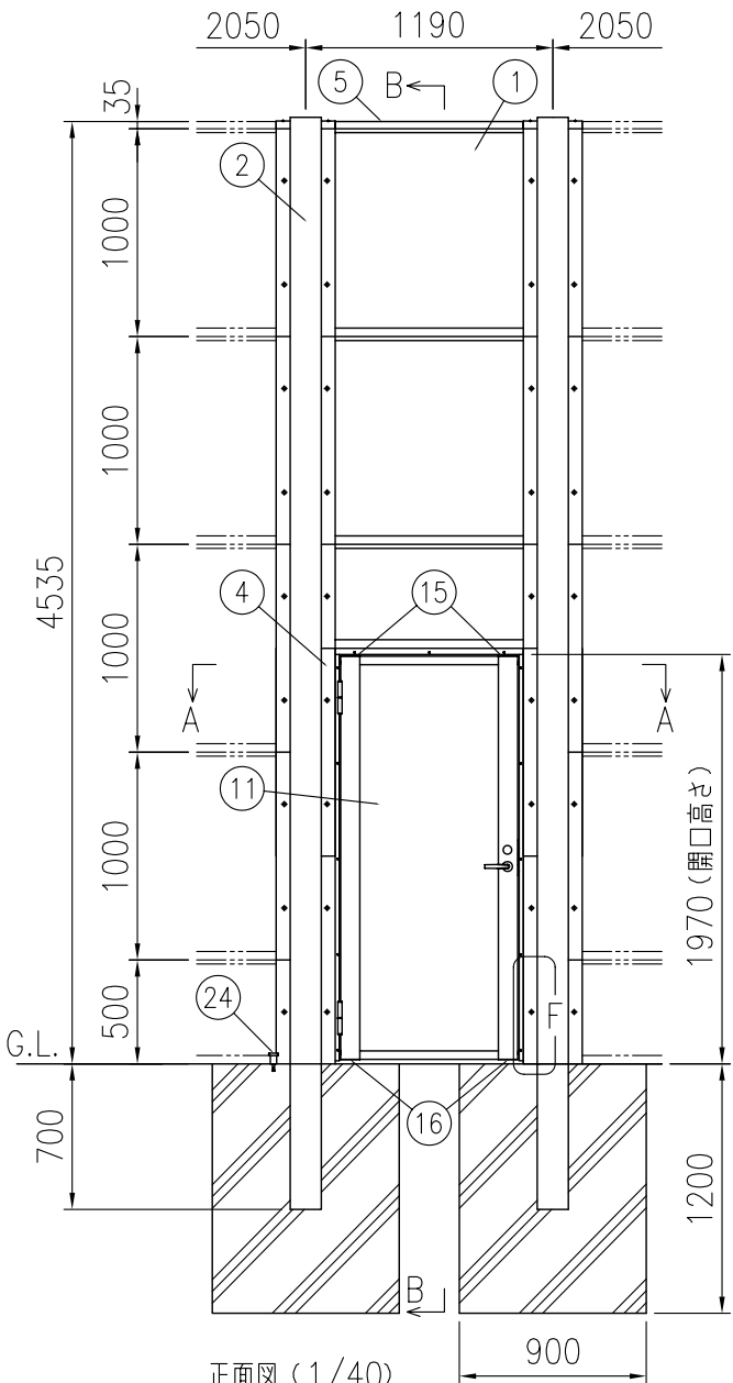
正面図 (1/40)
