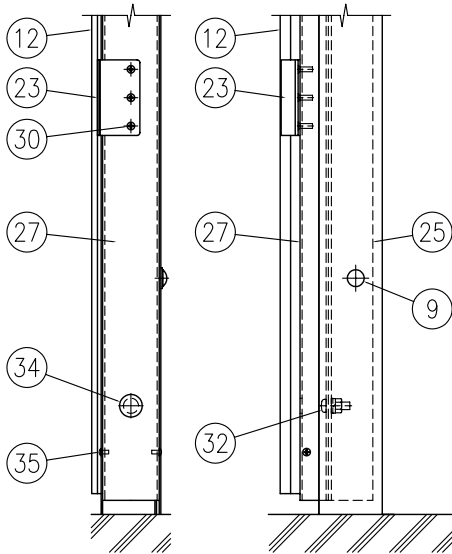
F部側面詳細図 (1/8)
