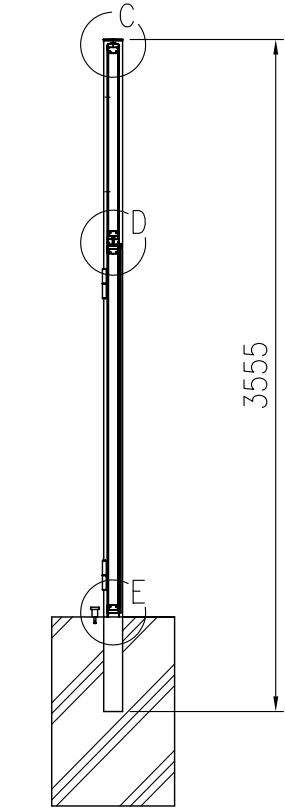
B-B 断面図 (1/40)
