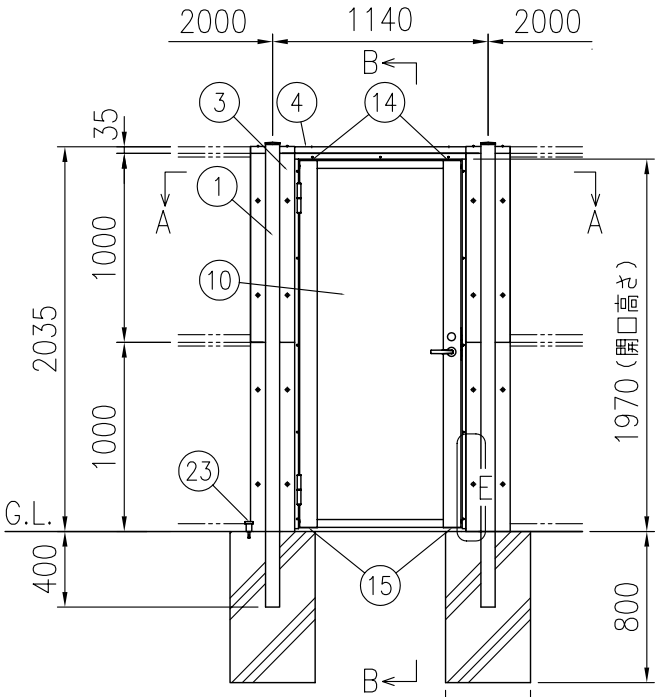
正面図 (1/40) 注) 基礎の大きさは参考寸法です。 注) くぐり戸仕様です。
