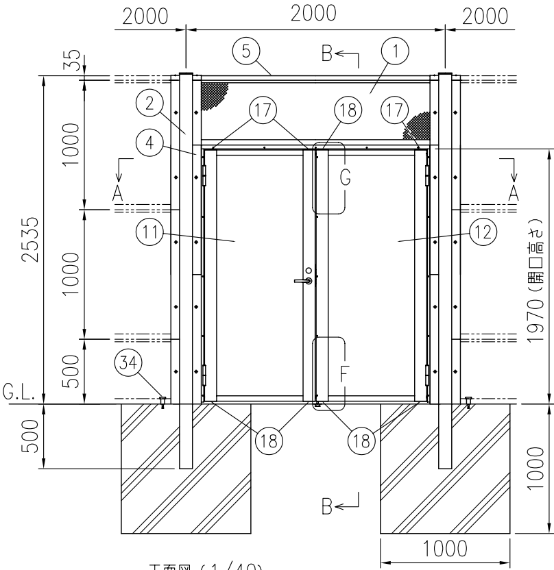
正面図 (1/40) 注) 基礎の大きさは参考寸法です。
