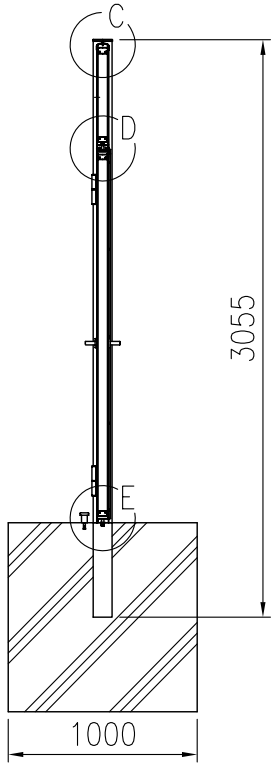
B-B 断面図 (1/40)
