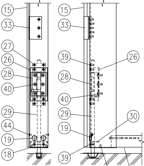
F部側面詳細図 (1/8) F部詳細図 (1/8)
