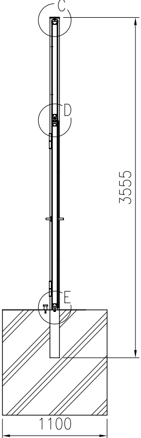
B-B 断面図 (1/40)
