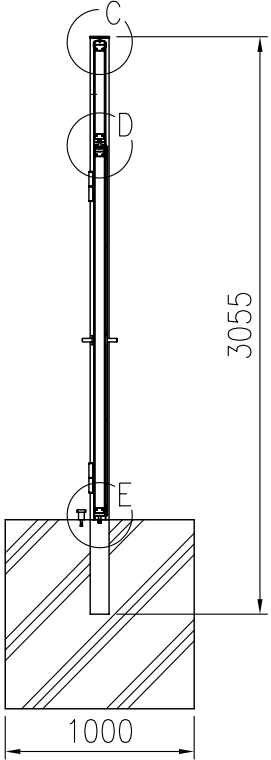
B-B 断面図 (1/40)
