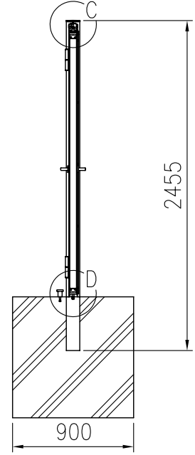
B-B 断面図 (1/40)
