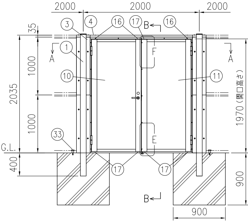
正面図 (1/40) 注) 基礎の大きさは参考寸法です。 注) くぐり戸仕様です。
