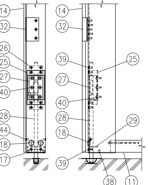
E部側面詳細図 (1/8) E部詳細図 (1/8) ※ 門扉パネル (受側) のE部とF部は上下対称
