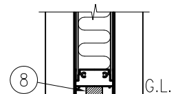
F部 詳細図 (1/8)
