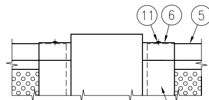
B部 詳細図 (1/8)
