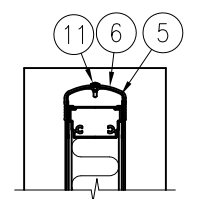
E部 詳細図 (1/8)
