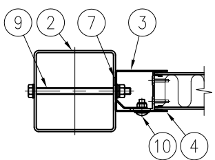
C-C断面図 (1/8)
