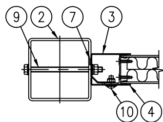
C-C 断面図 (1/8)
