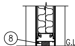
F部 詳細図 (1/8)
