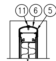
E部 詳細図 (1/8)
