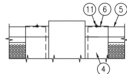
B部 詳細図 (1/8)
