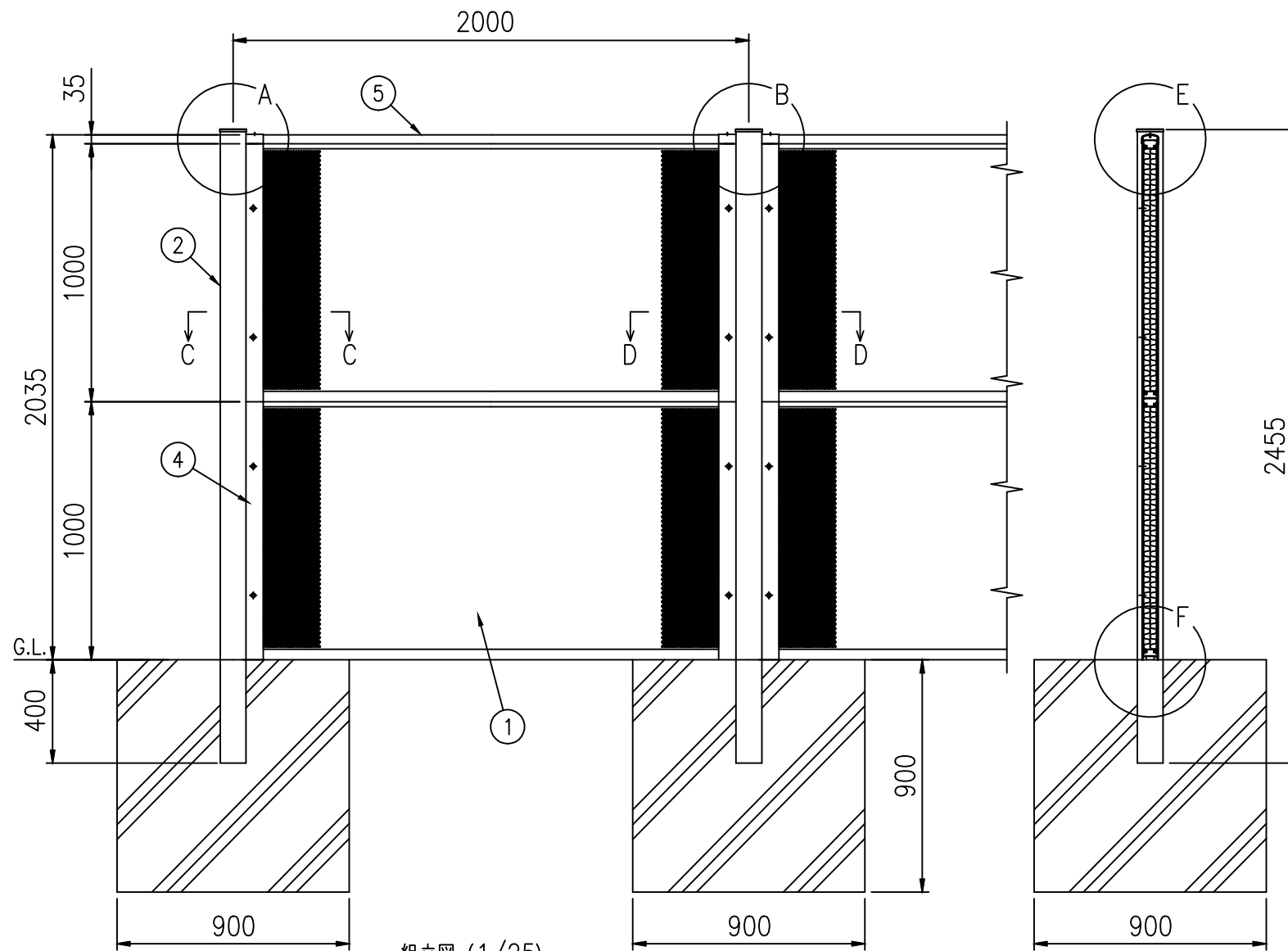
組立図 (1/25)
