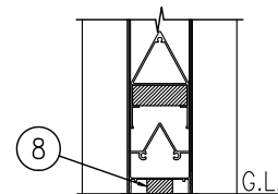
F部 詳細図 (1/5)
