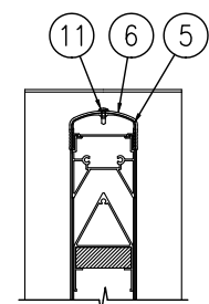
E部 詳細図 (1/8)
