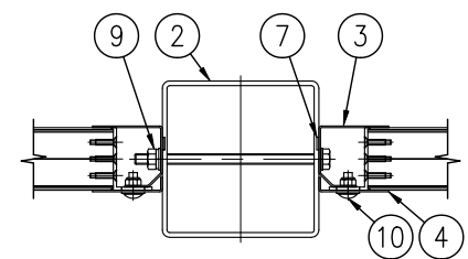
D-D 断面図 (1/8)
