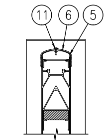
E部 詳細図 (1/8)
