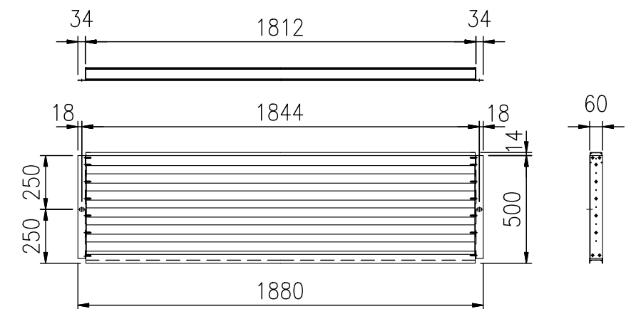
パネル H0.5m 詳細図 (1/25)
