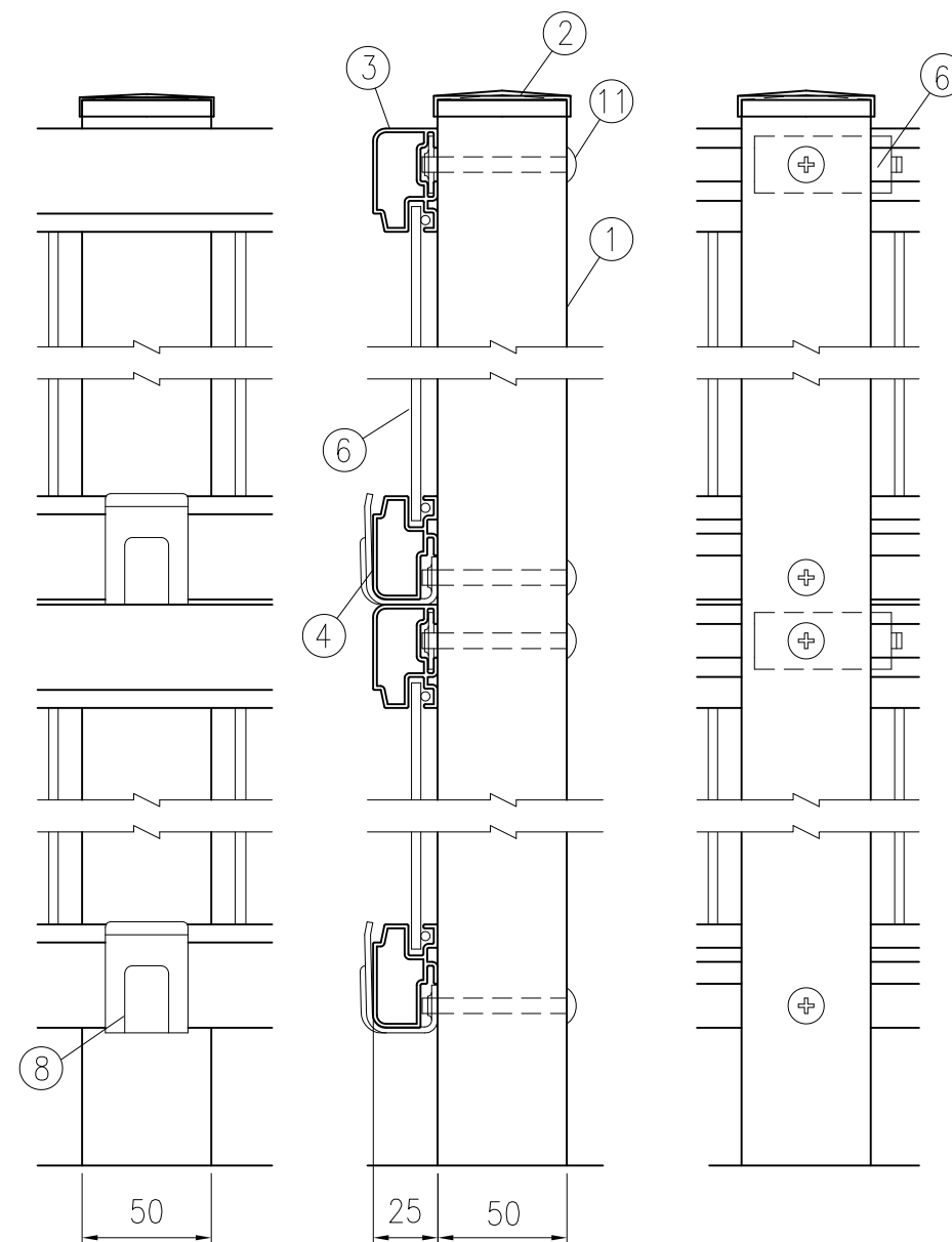
取付部詳細図 (1/3)
