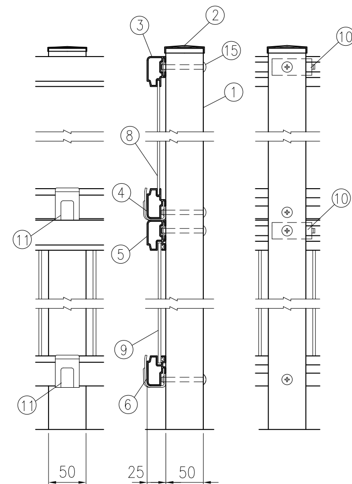
取付部詳細図 (1/5)
