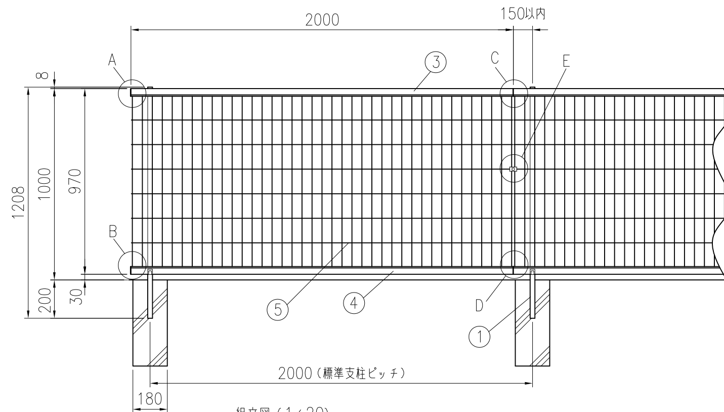
組立図 (1/20) 注) 基礎の大きさは、参考寸法です。
