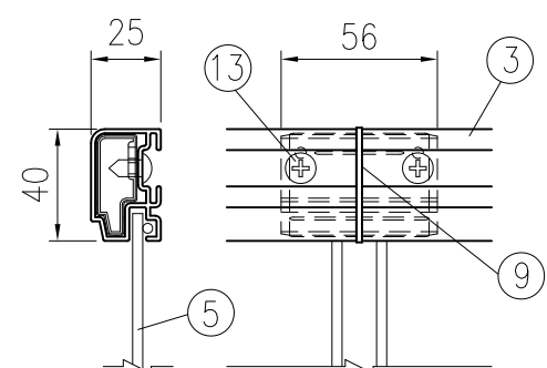
C部詳細図 (1/3)
