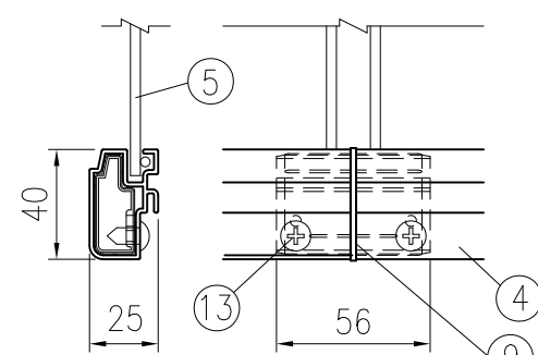
D部詳細図 (1/3)
